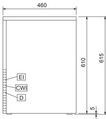
Zij aanzicht
